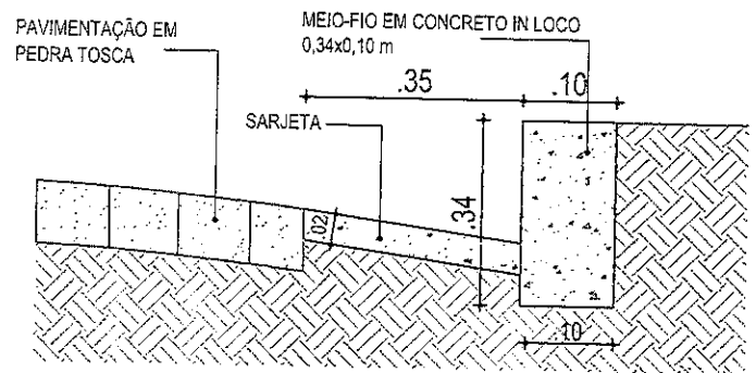
02 | DETALHE 02 - MEIO FIO CONJUGADO COM SARJETA ESC.: S/E
