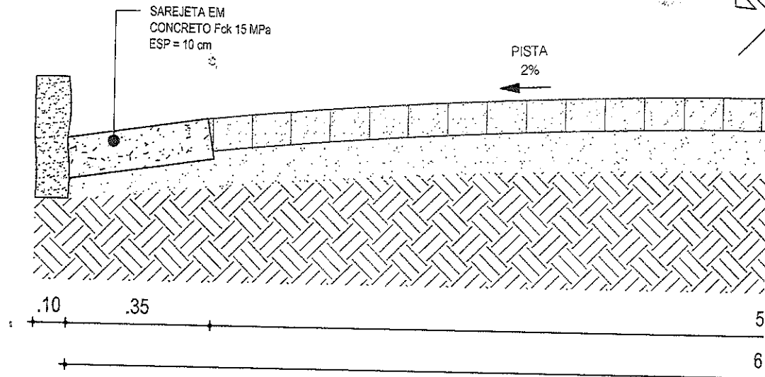
01 | SEÇÃO TIPO DE PAVIMENTAÇÃO ESC.: S/E
