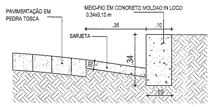
02 | DETALHE - MEIO FIO CONJUGADO COM SARJETA ESC.: S/E
