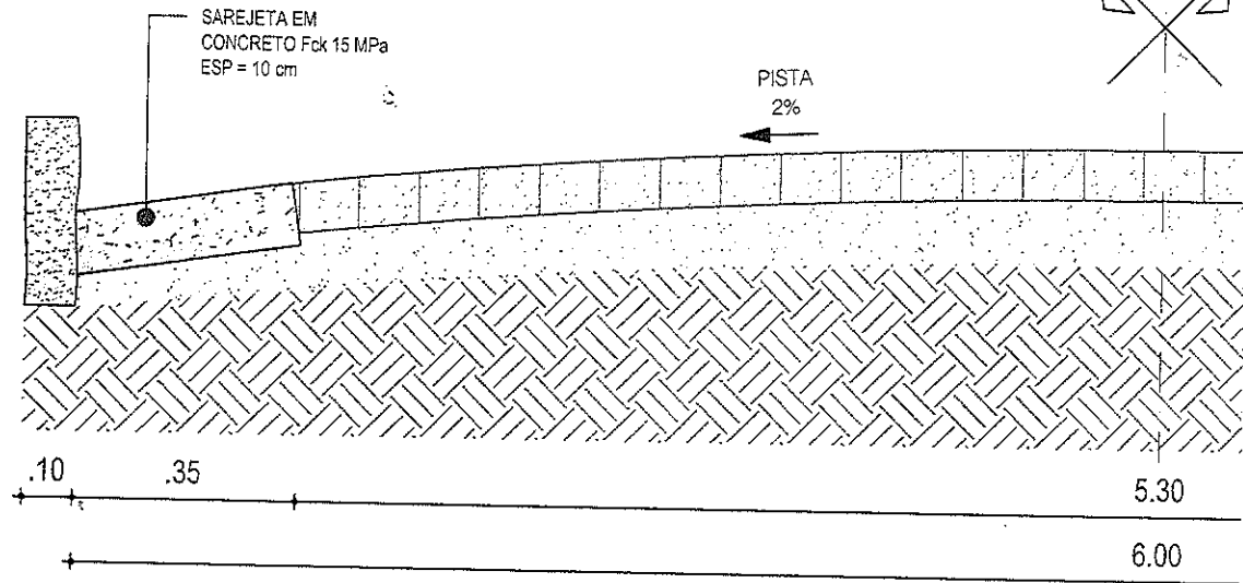
01 | SEÇÃO TIPO DE PAVIMENTAÇÃO ESC.: S/E
