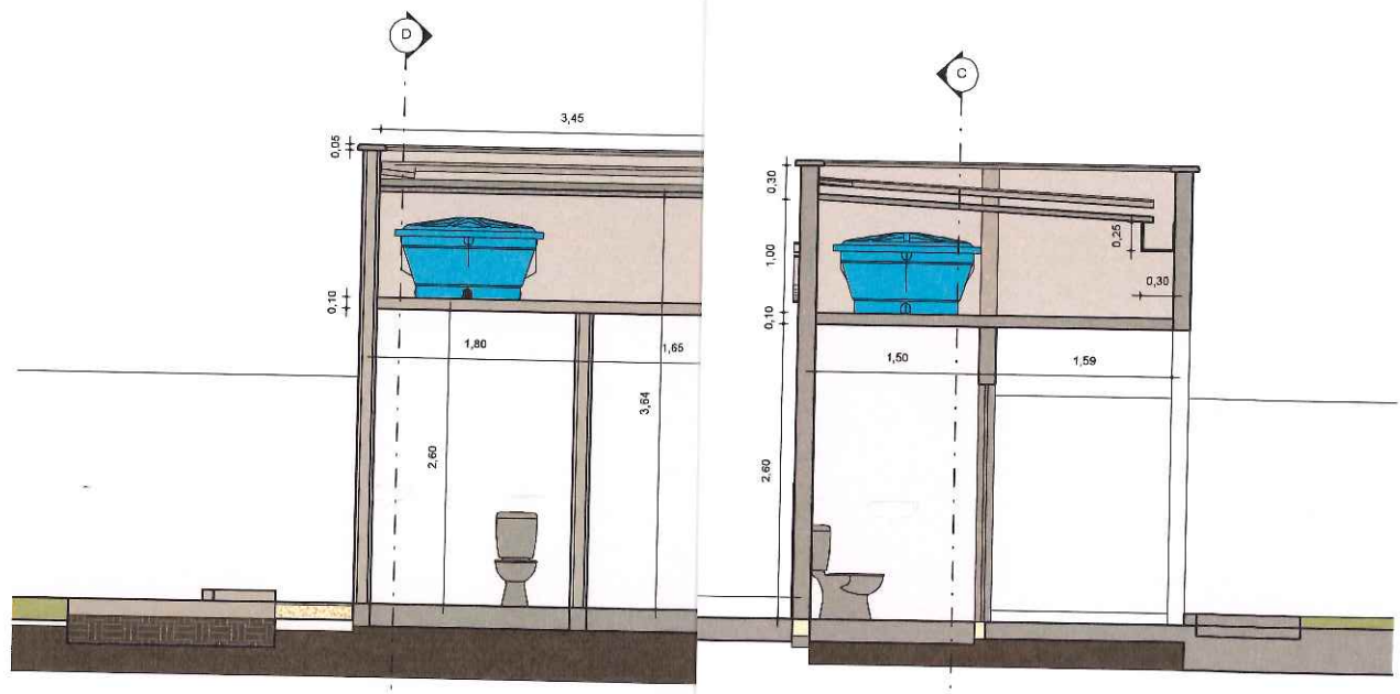
3 CORTE CC Escala: 1 : 25
